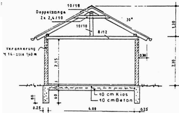
Querschnitt
