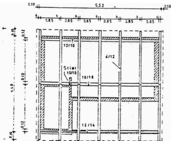
Sparrenlage (zugfest verankern)
