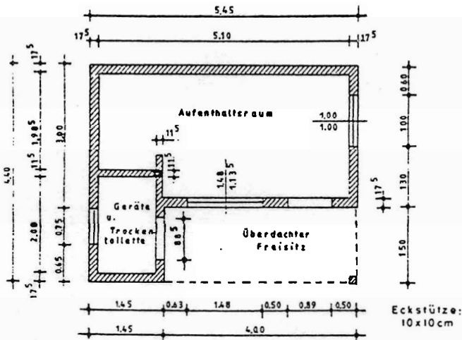
Grundriß
